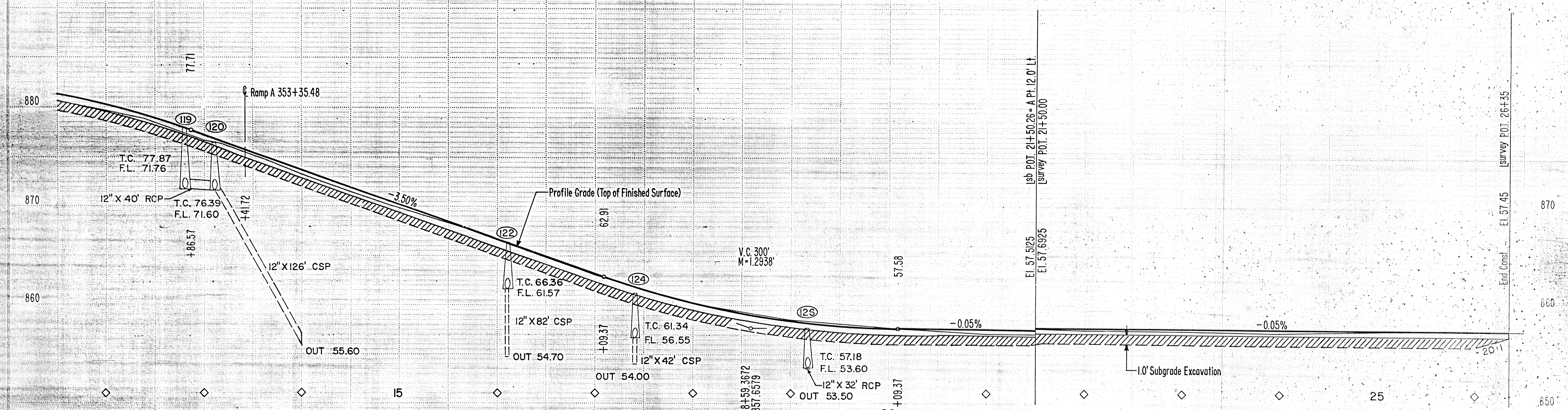
LSB STA. P.O.T. 92+49.01 — SURVEY STA. P.O.T. 26+35.00 PROFILE
