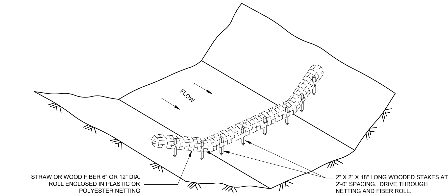
BIO-ROLLS N.T.S.
